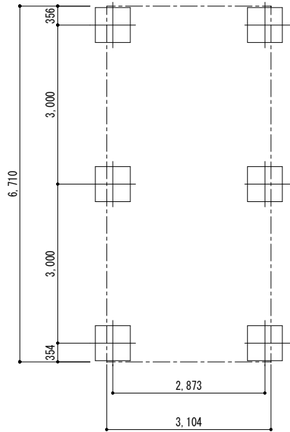
■ 基礎配置図
